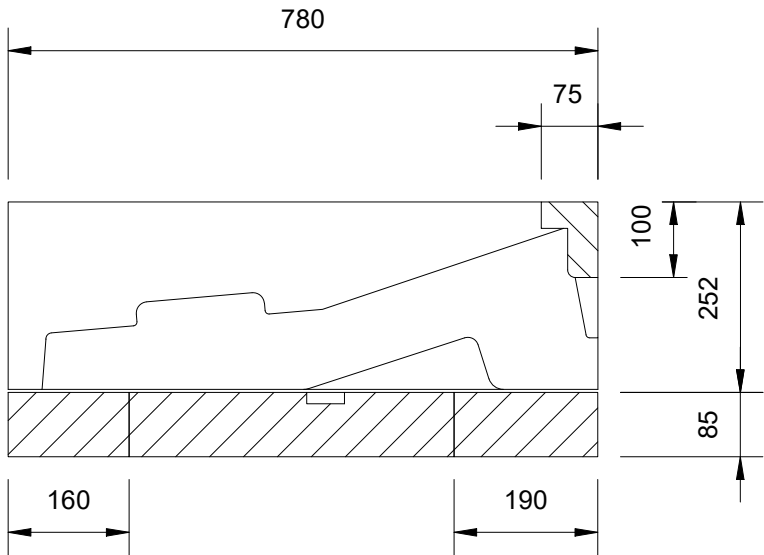
SECTION B-B : D9-215 CONSOLE FOAM ( SCALE 1 : 10 )
